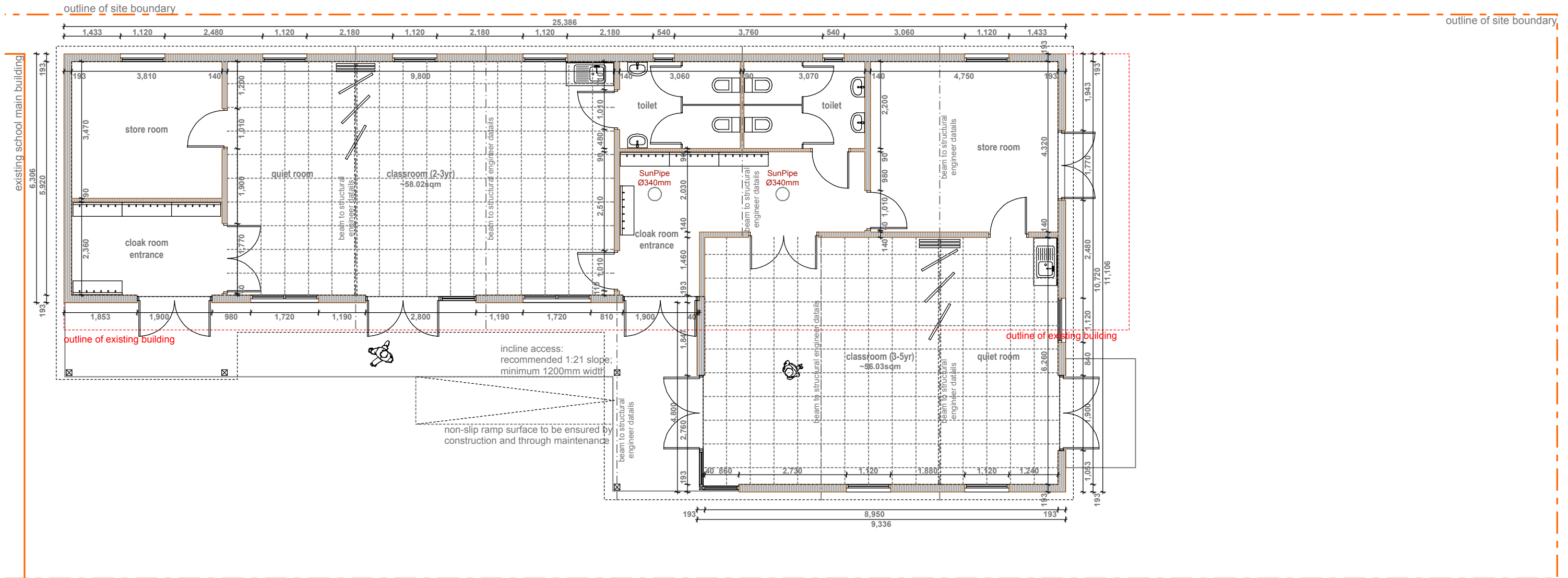
Plan Layout & Site Plan 1:100
